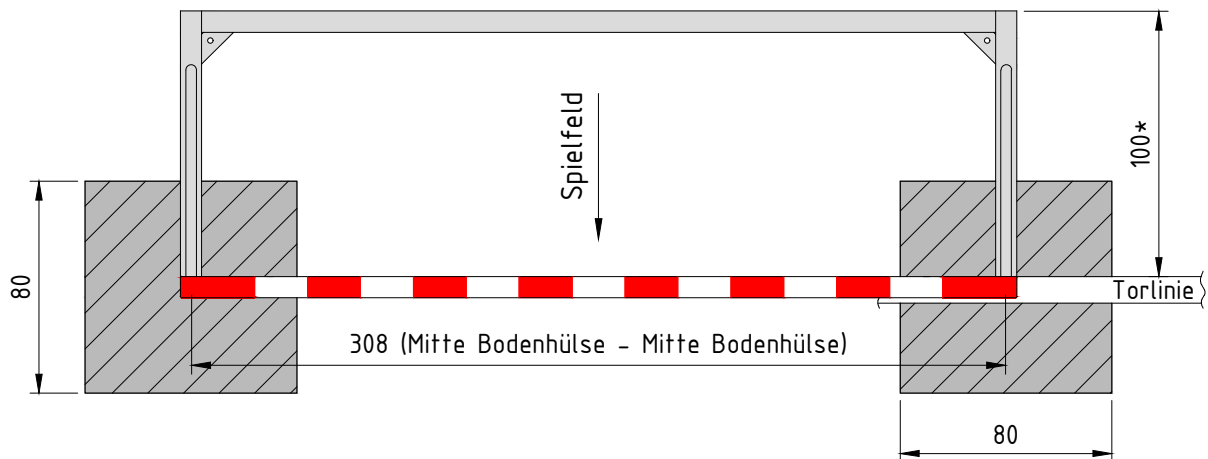
*Abb. Handballtor "Competition" mit Bodenrahmen
